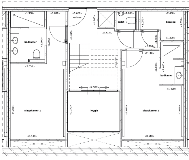
Plattegrond verdieping 03 1:50
