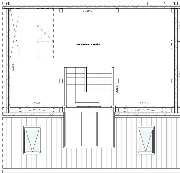
Plattegrond verdieping 04 1:50
